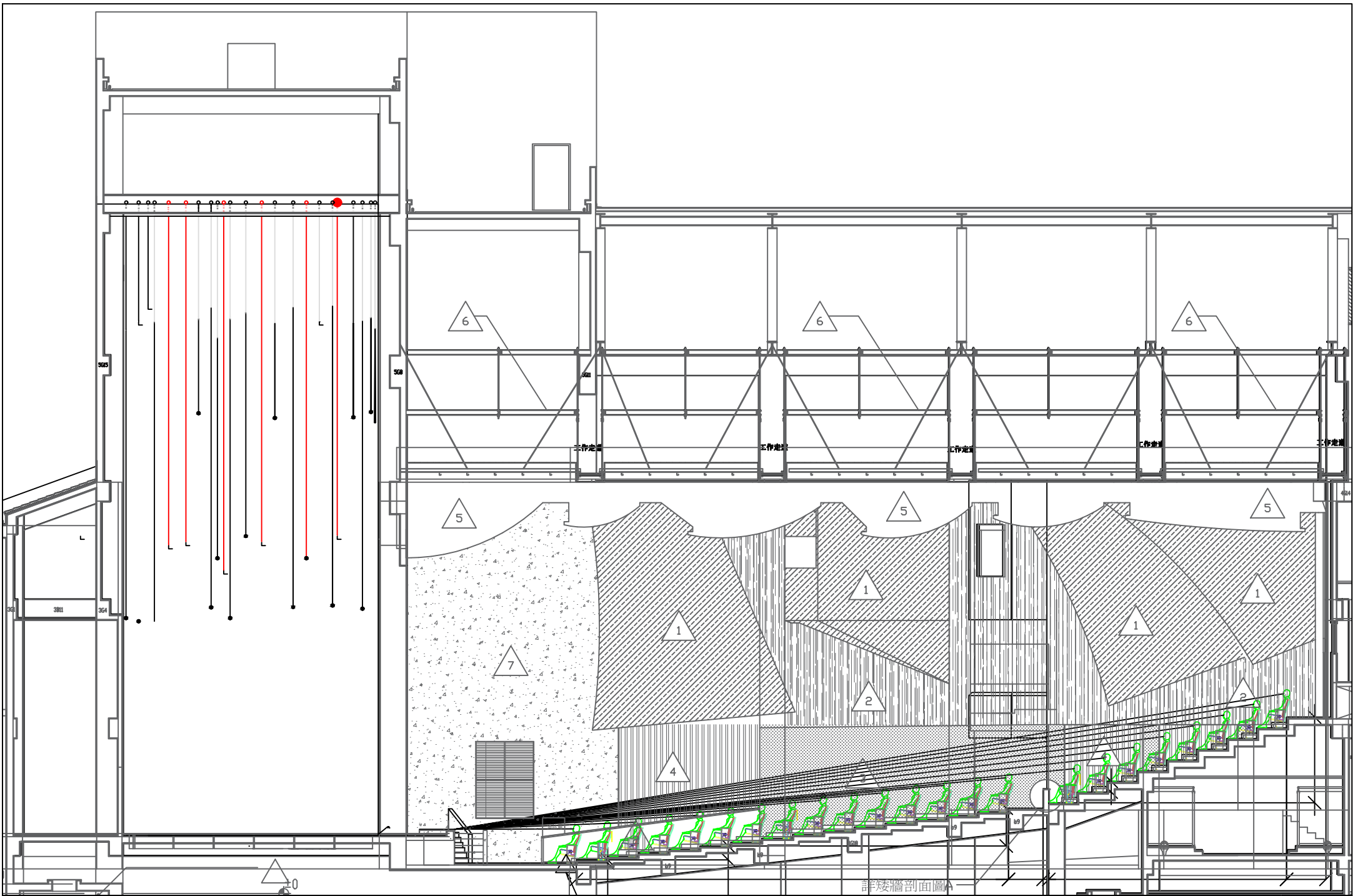
台南歸仁文化中心舞台吊桿剖面圖 比例：1:1 資料更新：2022/07/05
